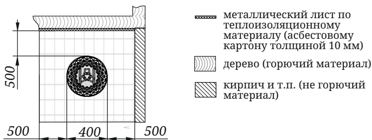
Рисунок 3. Монтаж площадки-постамента
